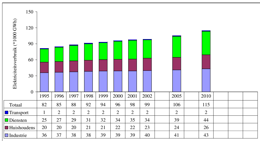
Figuur 1 Elektriciteitgebruik (in TWh) in Nederland in de periode 1995-2010. Bronnen: Historisch CBS (2004), prognose (ECN, RIVM, 2002).
